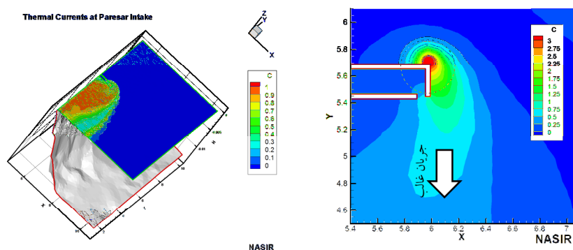
شکل ۱۲- دمای میانگین در اطراف خروجی نیروگاه پره سردر شرایط باد و بدون جریان غالب (واحدهای مختصات بر حسب کیلومتر می‌باشند)
