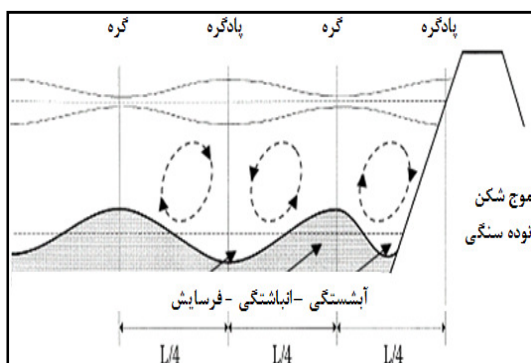
شکل ۲- اثر متقابل موج و سازه
