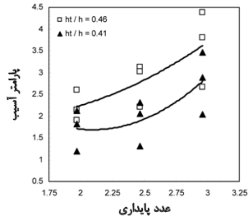
شکل ۶- میزان آسیب پنجه موج شکن ( \alpha = 1:0.66 )
