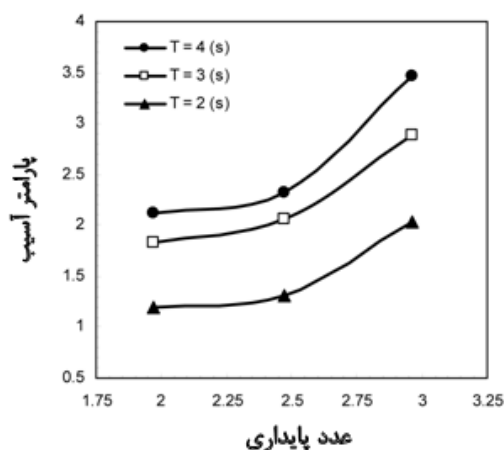
شکل ۴- میزان آسیب پنجه موج شکن ( h = 54 (cm), \alpha = 1:0 +/۶۶)
