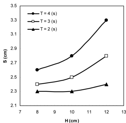
شکل ۳- میزان آبشستگی پنجه موج شکن ( h = 54 (cm), \alpha = 1:0 +/۶۶)
