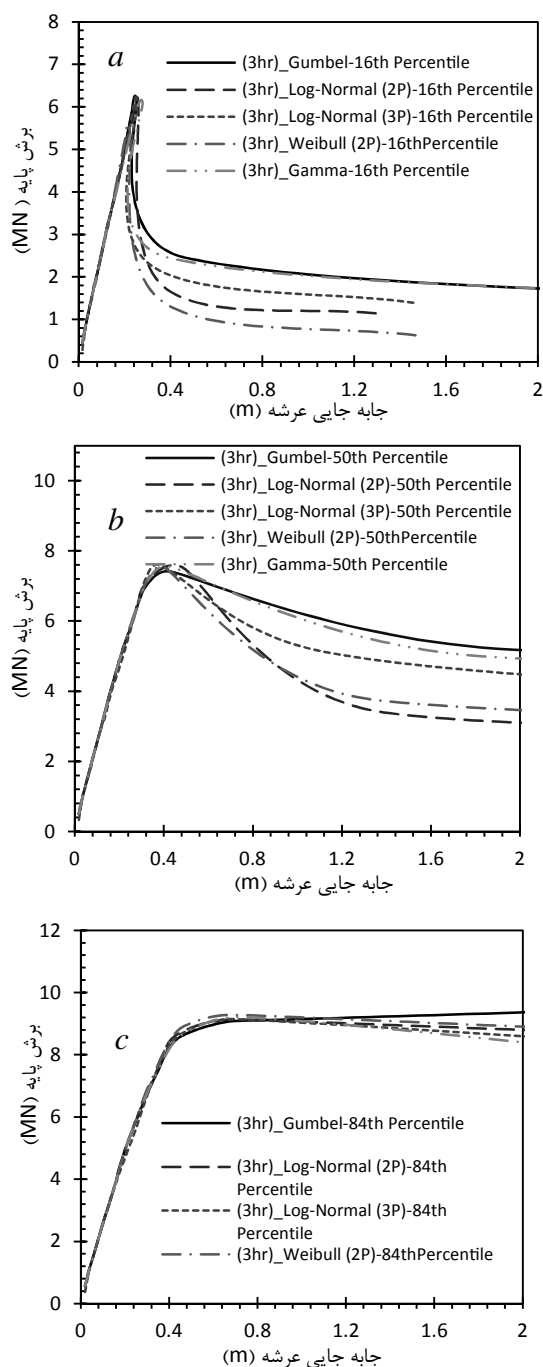
شکل ۶- منحنی‌های ظرفیت استخراج شده با رویکرد تحلیلی بر روی امواج تصادفی بلندمدت ۳ ساعته. (a) صدک ۱۶٪ (b) صدک ۵۰٪ و (c) صدک ۸۴٪.
