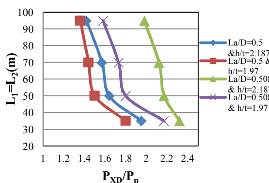
شکل ۱۲- نمودار رابطه بین فاصله کمانش گیرها با فشار گذر نسبی برای \frac{D}{t} = 15
