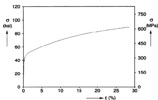
شکل ۴- منحنی تنش-کرنش اصلاح شده [۸، ۷، ۱۲] (n=12) Ramberg-Osgood
