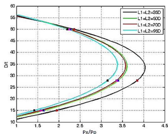
شکل ۱۴- نمودار تغییرات فشار گذر نسبی نسبت به \frac{D}{t} برای \frac{L_a}{D} = 0.5 و \frac{h}{t} = 2.187
