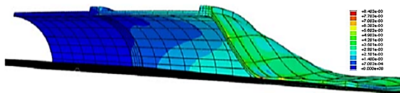
شکل ۶- انتشار کمانش شبه استاتیکی
