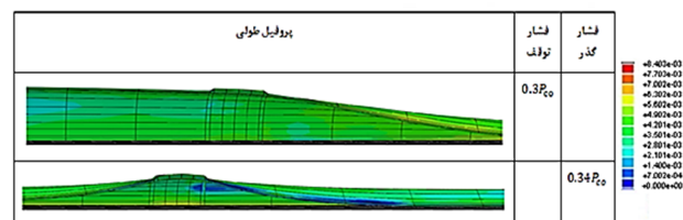
شکل ۱۳- تغییر شکل مقطع طولی زمانی که کمانش منتشر شده متوقف شده یا از کمانش گیر عبور می کند برای \frac{D}{t} = 50
