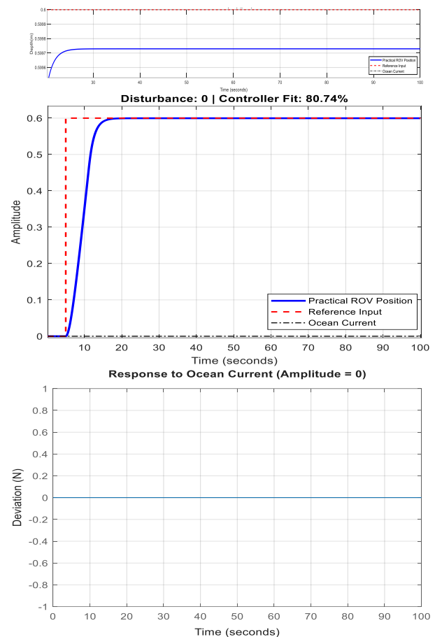
شکل ۲۴- ردیابی مرجع کنترلر بدون حضور اغتشاش جریان
