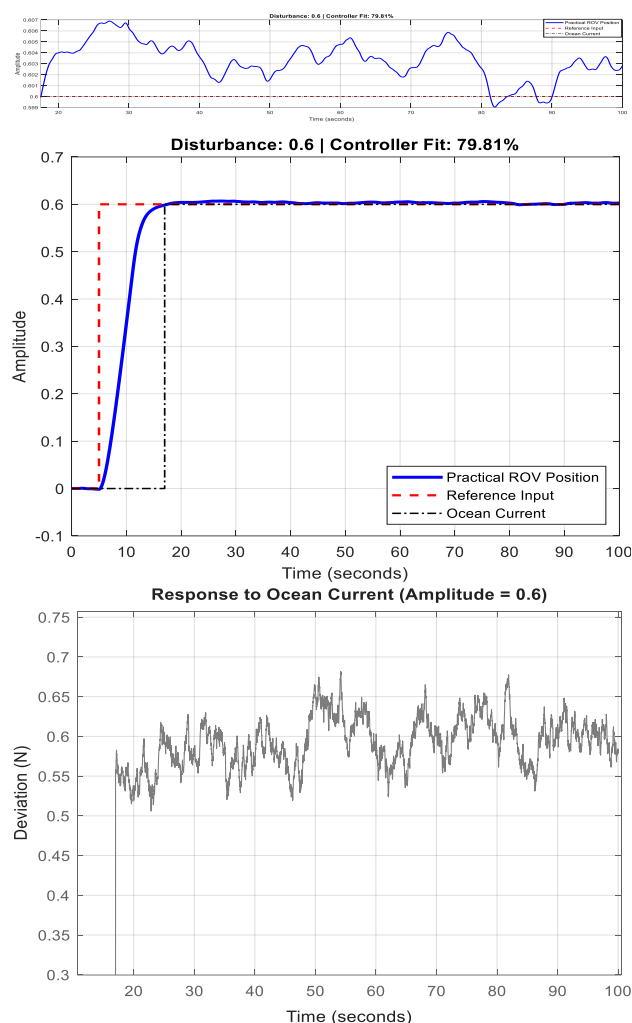
شکل ۲۴- ردیابی مرجع کنترلر در حضور اغتشاش ۰/۶ نیوتن
