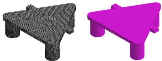
شکل ۴- مش‌بندی پلتفرم
