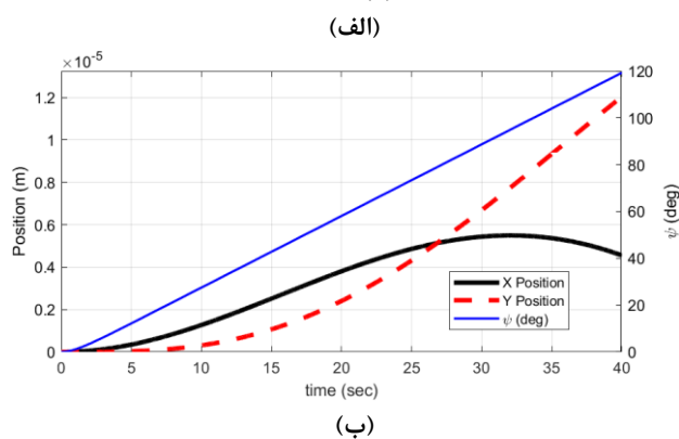
شکل ۱۰- نتایج شبیه‌سازی سناریو ۴ صحت عملکرد مدل دینامیکی. الف) نمایش انیمیشن حرکت شناور. ب) حرکت شناور در راستای X, Y و \psi .
