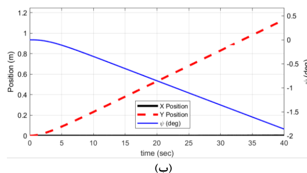
شکل ۹- نتایج شبیه‌سازی سناریو ۳ صحت عملکرد مدل دینامیکی. الف) نمایش انیمیشن حرکت شناور. ب) حرکت شناور در راستای X, Y و \psi .
