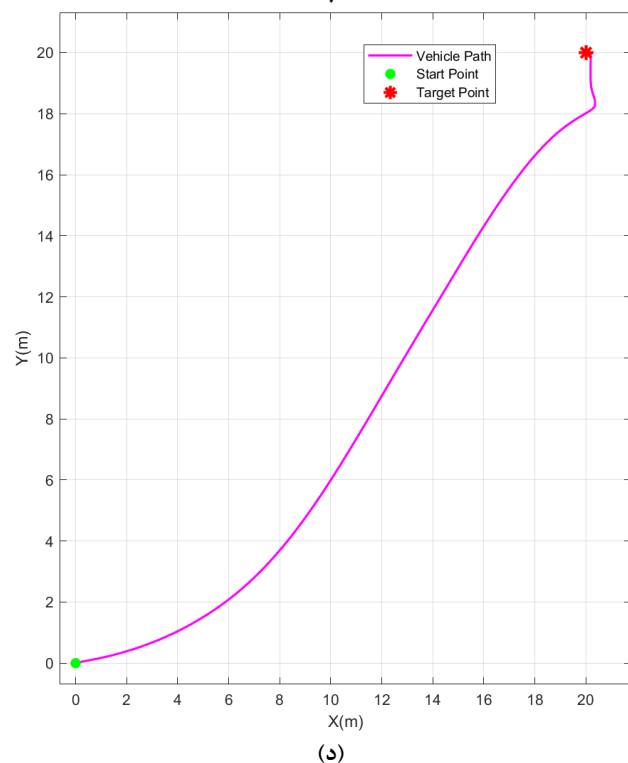
شکل ۱۴- نتایج شبیه سازی سناریو ۴ سیستم موقعیت یابی پویا.
