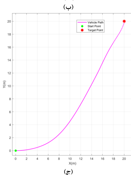
شکل ۱۱- نتایج شبیه‌سازی سناریو ۱ سیستم موقعیت‌یابی پویا. (الف) نمایش انیمیشن موقعیت شناور. (ب) حرکت شناور در راستای X, Y, \psi . (ج) مسیر حرکت شناور در محور X-Y در طول شبیه‌سازی.
