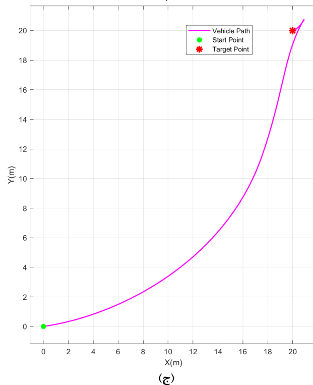
شکل ۱۳- نتایج شبیه سازی سناریو ۳ سیستم موقعیت یابی پویا.
