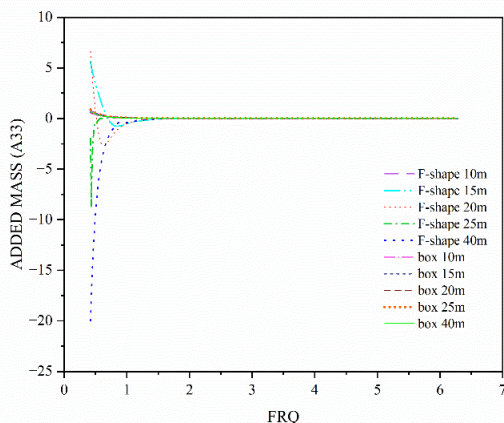
شکل ۲۱- تغییرات ضریب جرم افزوده در راستای قائم دو مقطع موج شکن شناور مستطیلی و اف شکل در طول های مختلف
