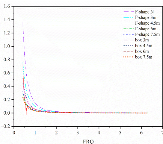
شکل ۹- تغییرات ضریب جرم افزوده در راستای قائم بر حسب فرکانس در اعماق مختلف فرورفت موج شکن
