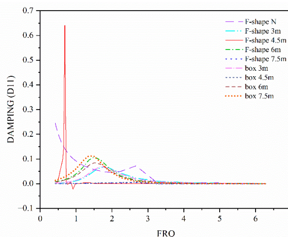
شکل ۸- ضریب میرایی هیدرودینامیکی (D11) در راستای افقی دو مقطع موج شکن شناور مستطیلی و اف شکل در اعماق مختلف فرورفت
