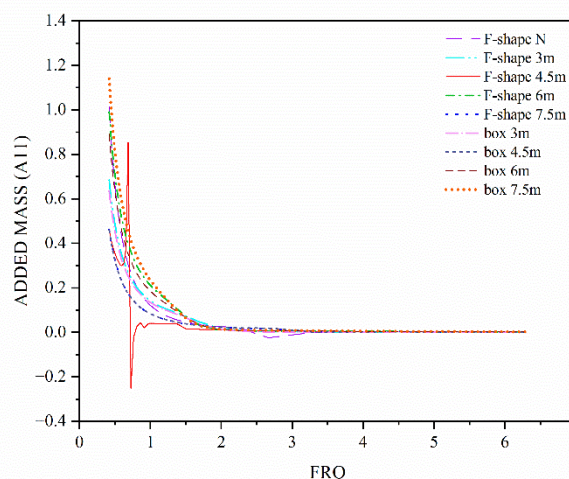
شکل ۷- تغییرات ضریب جرم افزوده (A11) در راستای افقی دو مقطع موج شکن شناور مستطیلی و اف شکل در اعماق مختلف فرورفت
