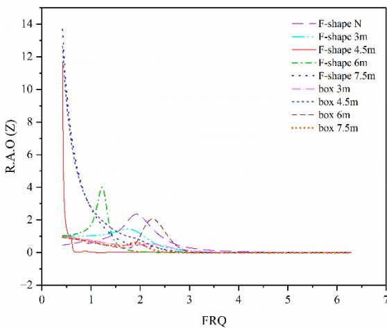
شکل ۱۴- پاسخ دینامیکی سازه‌های شناور با مقاطع اف شکل و مستطیلی تحت تاثیر امواج منظم را در جهت قائم
