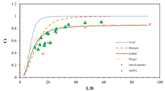
شکل ۳- داده‌های آزمایشگاهی Koutandos و همکاران (۲۰۰۵) برای موج‌شکن ثابت در مقایسه با مدل عددی AQWA، امواج منظم ( H=2\text{m} ) [21-24]، B=2\text{m}
