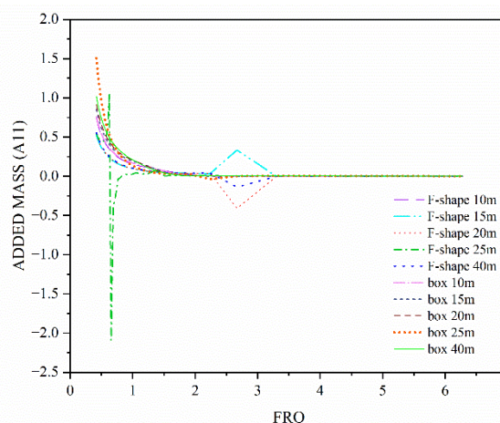
شکل ۱۹- تغییرات ضریب جرم افزوده (A11) در راستای افقی دو مقطع موج شکن شناور مستطیلی و اف شکل در طول های مختلف
