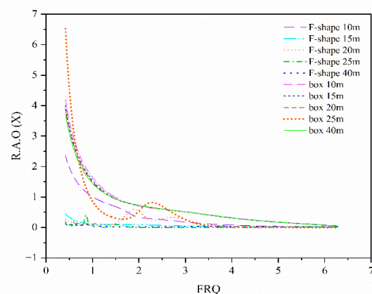
شکل ۲۵- پاسخ دینامیکی سازه‌های شناور با مقاطع اف شکل و مستطیلی تحت تاثیر امواج منظم را در جهت افقی
