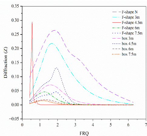
شکل ۵- تغییرات نیروی قائم دو نوع موج‌شکن شناور با مقاطع مستطیلی و اف شکل در اعماق مختلف فرو رفت
