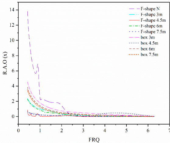
شکل ۱۳- پاسخ دینامیکی سازه‌های شناور با مقاطع اف شکل و مستطیلی تحت تاثیر امواج منظم را در جهت افقی
