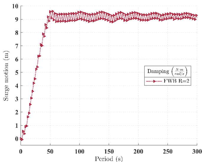
شکل ۲۶: حرکت سرچ موجشکن در پریود ۵ ثانیه با مبدل ۲ متر و چیدمان ۱
