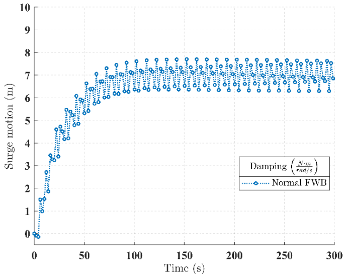
شکل ۲۰- حرکت سرج موج‌شکن در پریود ۵ ثانیه بدون مبدل
