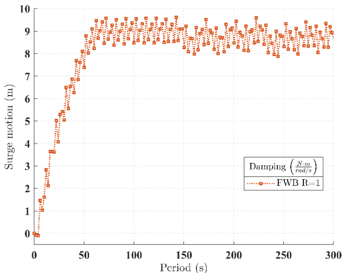
شکل ۲۱- حرکت سرج موج‌شکن در پریود ۵ ثانیه با مبدل ۱ متر و چیدمان ۱
