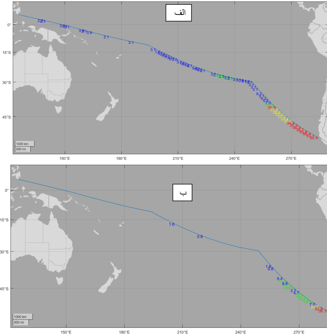
شکل ۴-الف- درصد سرعت باد بالای ۲۰ گره و ب- بالای ۲۵ گره در مسیر دریانوردی از تنگه سرنگانی به جزیره ایستر و تنگه ماژلان در مورخه ۱۴۰۲/۰۹/۱۰ که بهترین وضعیت جوی در این مسیر حاکم است (توضیحات رنگ بندی اعداد روی نقشه در متن آورده شده است).
