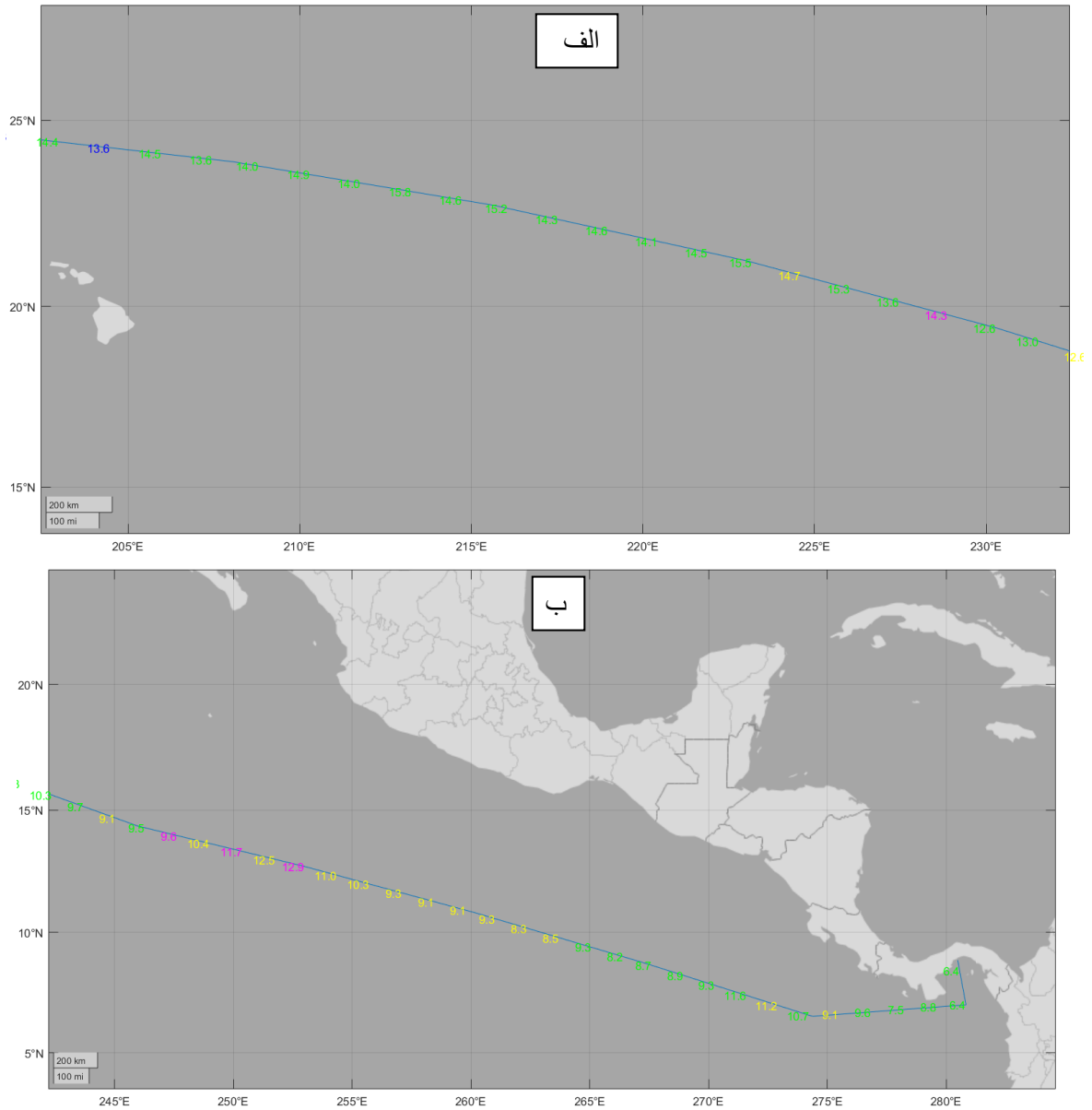
شکل. میانگین سرعت باد در مسیر یوکوهاما، هاوایی، پاناما (توضیحات رنگ بندی اعداد روی نقشه در متن آورده شده است)، الف- در بخش جزیره هاوایی، ب- بخش انتهایی در مورخه ۲۰۲۳/۰۸/۰۱ معادل با ۱۴۰۲/۰۵/۱۰.
