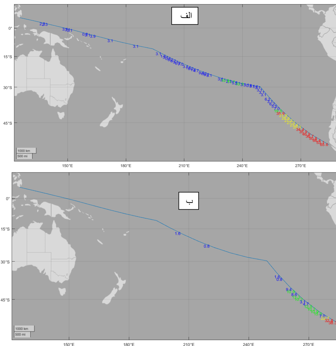
شکل ۴- الف- درصد سرعت باد بالای ۲۰ گره و ب- بالای ۲۵ گره در مسیر دریانوردی از تنگه سرنگانی به جزیره ایستر و تنگه ماژلان در مورخه ۲۰۲۳/۱۲/۰۱ معادل با ۱۴۰۲/۰۹/۱۰ که بهترین وضعیت جوی در این مسیر حاکم است (توضیحات رنگ بندی اعداد روی نقشه در متن آورده شده است).
