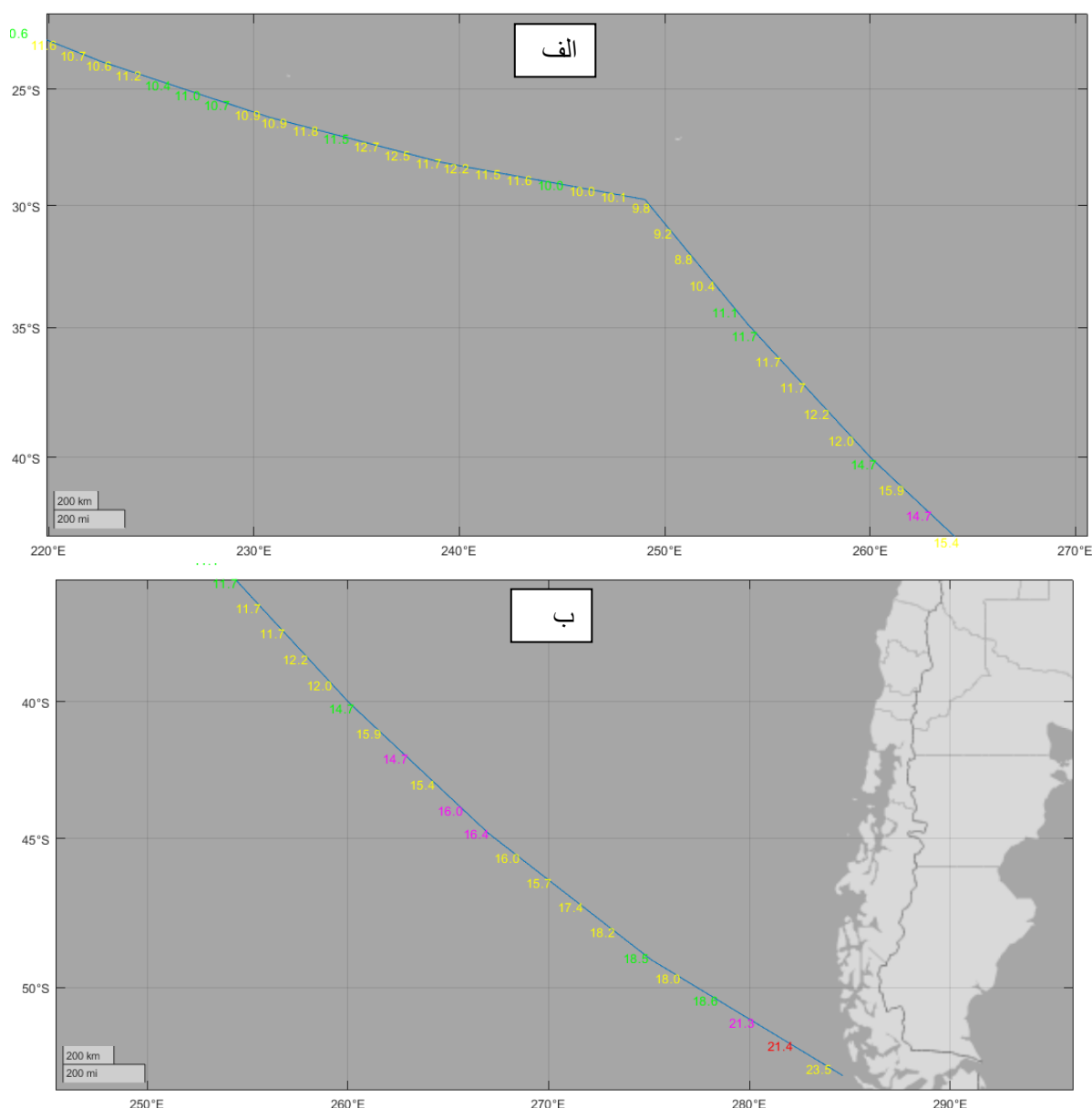
شکل ۲-۳- مسیر از سرنگانی به جزیره ایستر و بندر والپرایزو و تنگه ماژلان (توضیحات رنگ بندی اعداد روی نقشه در متن آورده شده است)، الف- در جزیره ایستر، ب- بخش انتهایی مسیر در مورخه ۲۰۲۳/۱۲/۰۱ معادل با ۱۴۰۲/۰۹/۱۰.
