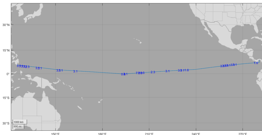
شکل ۴-۳- مسیر بندر یوکوهاما، جزایر هاوایی و کانال پاناما استوا و کانال پاناما در مورخه ۲۰۲۳/۱۱/۱۰ معادل ۱۴۰۲/۰۸/۱۹ مطابق با بدترین وضعیت جوی (توضیحات رنگ بندی اعداد روی نقشه در متن آورده شده است)
