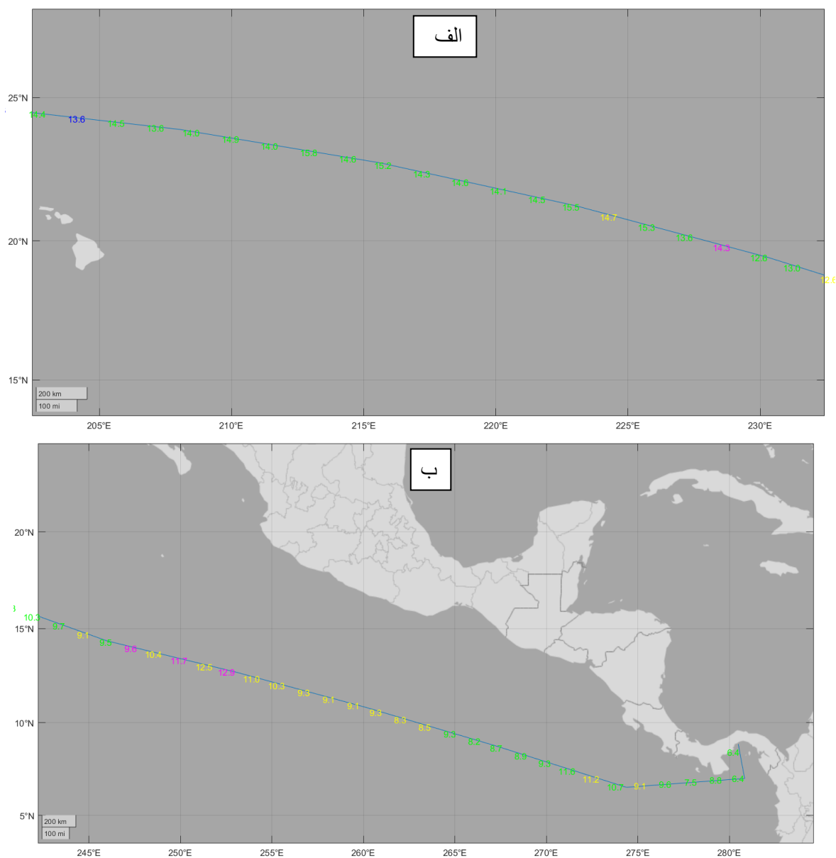
شکل. میانگین سرعت باد در مسیر یوکوهاما، هاوایی، پاناما (توضیحات رنگ بندی اعداد روی نقشه در متن آورده شده است)، الف - در بخش جزیره هاوایی، ب - بخش انتهایی در مورخه ۲۰۲۳/۰۸/۰۱ معادل با ۱۴۰۲/۰۵/۱۰.
