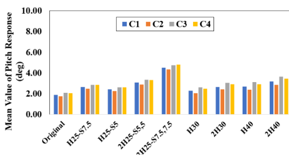
شکل ۱۸. میانگین پاسخ پیچ توربین بادی اصلاح شده با ورق های میراگر
