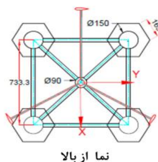
شکل ۳. هندسه بدنه توربین بادی چهار ستونه همراه با پانتونها، سمت چپ نما از بالا را نشان می دهد و سمت راست نما از روبرو [۱۲]
