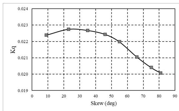
شکل ۱۰ نمودار ضريب گشتاور برحسب زاویه اسکيو در ضريب پيشروي ۰/۵
