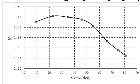
شکل ۹ نمودار ضريب تراست برحسب زاویه اسکيو در ضريب پيشروي ۰/۵
