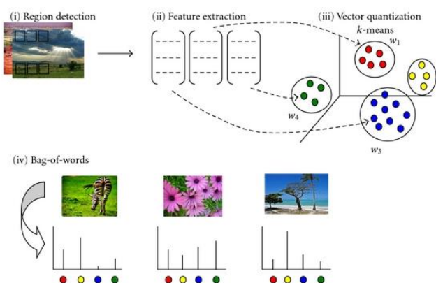
شکل ۴- فرآیند استخراج مشخصه بسته کلمات از تصاویر [۲۳]
