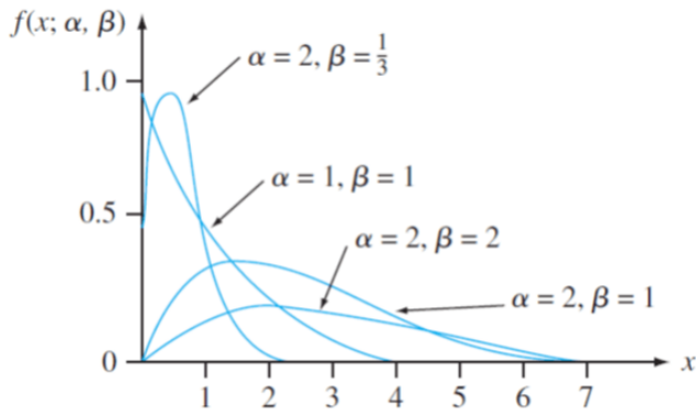
شکل ۳- نمایی از تابع توزیع گاما با پارامترهای متفاوت [۸]
