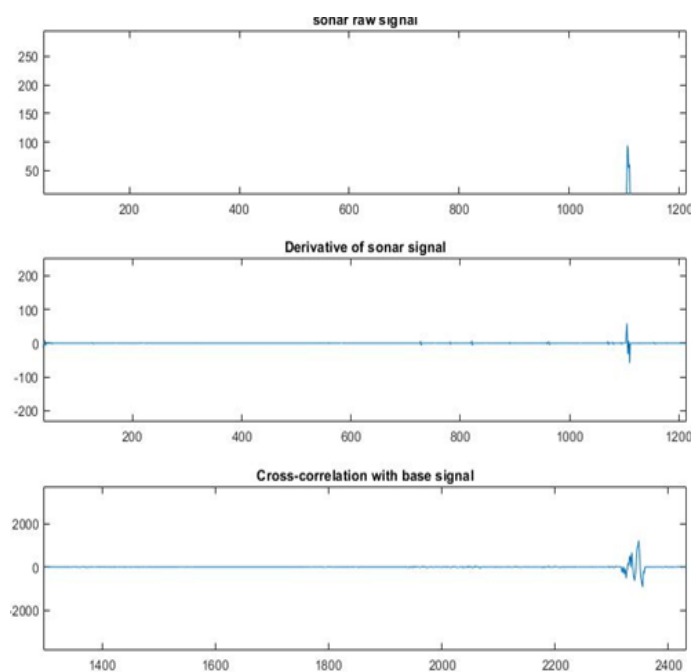
شکل ۱۲- نمایشی از مراحل تشخیص نقطه اکسترمم و ماسک گذاری در سیگنال سونار
