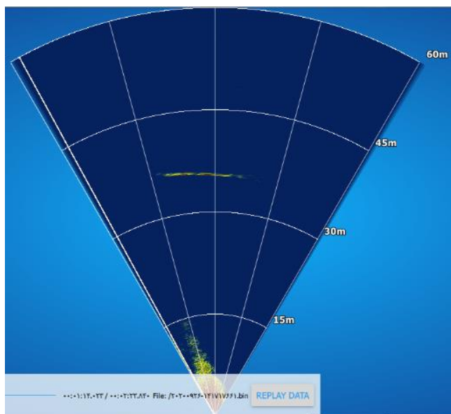
شکل ۵- بازخورد پژواک از اشیا و تشکیل تصویر آکوستیکی
