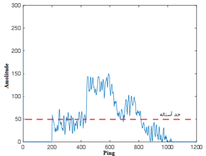
شکل ۱۰- استفاده از مفهوم حد آستانه برای حذف نویز پس‌زمینه محیط از پاکت اطلاعات سونار
