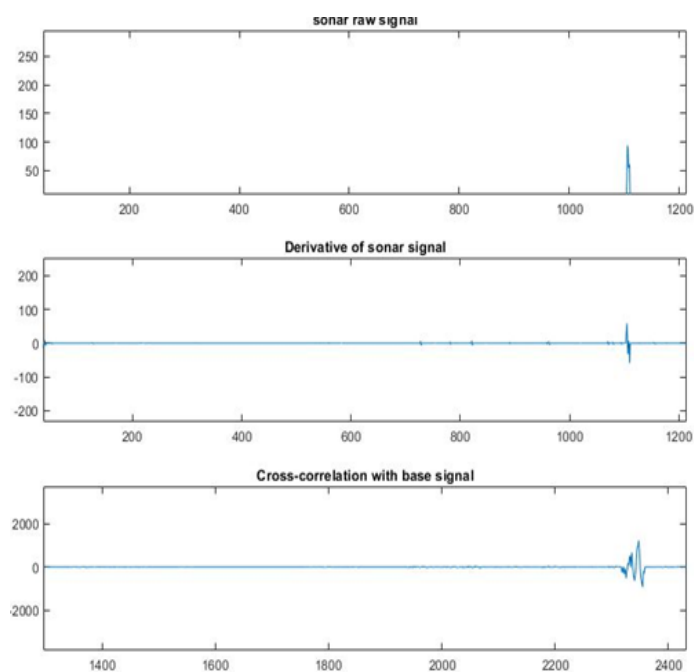
شکل ۱۲- نمایی از مراحل تشخیص نقطه اکسترمم و ماسک گذاری در سیگنال سونار
