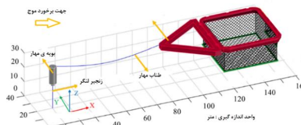
شکل ۵- قفس کشتی مانند تک مهاره [۲۶].
