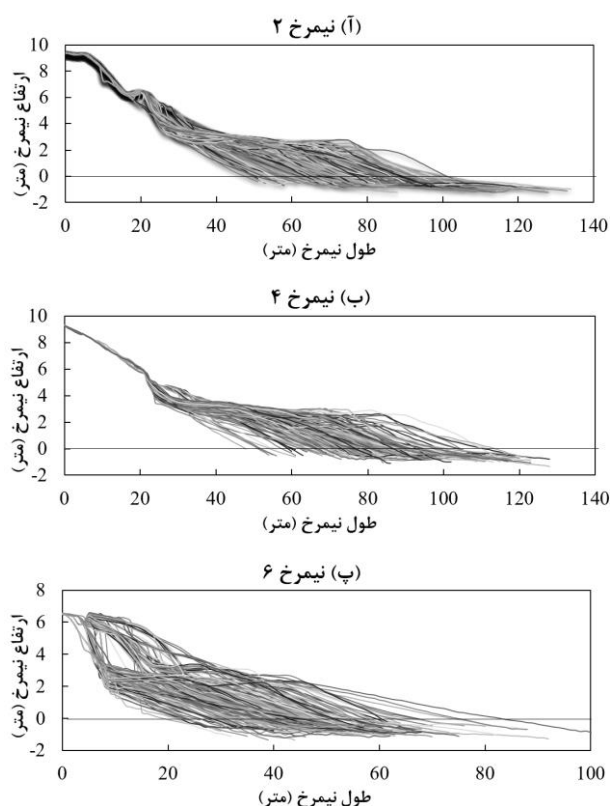
شکل ۲- نیمرخ‌های اندازه‌گیری شده از ساحل نارابین در بازه سال‌های ۲۰۰۶ تا ۲۰۱۹؛ آ. نیمرخ‌های شماره ۲؛ ب. نیمرخ‌های شماره ۴؛ پ.
