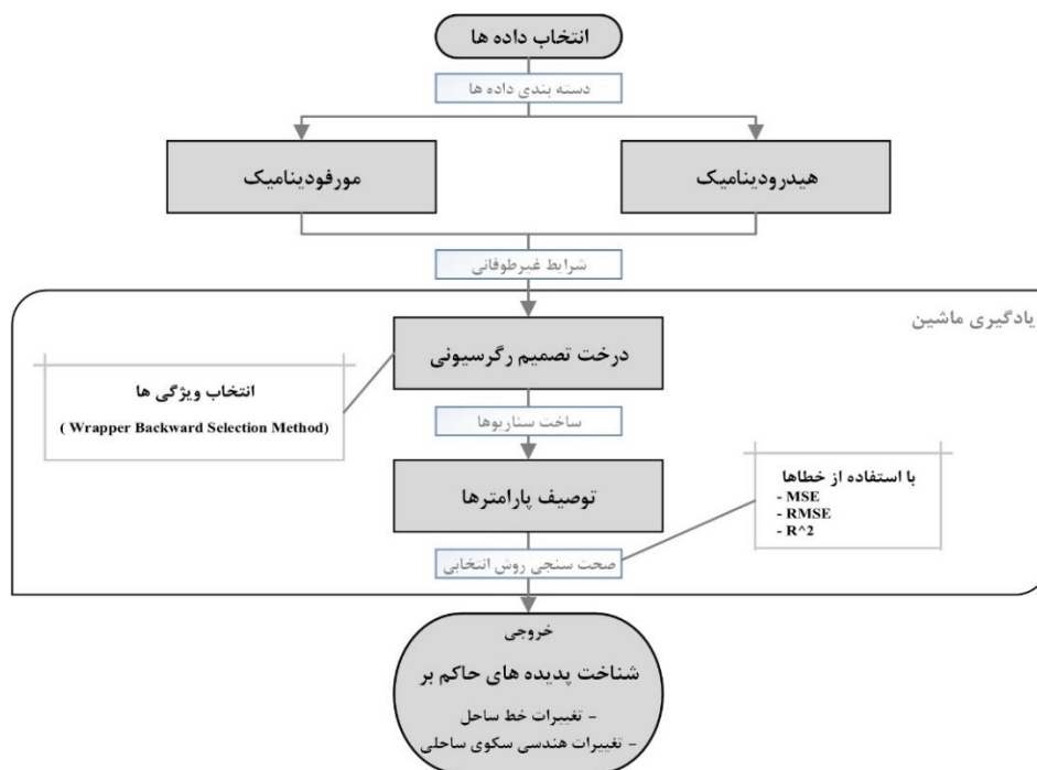
شکل ۷- فلوچارت روش انجام پژوهش
