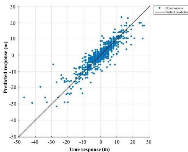
شکل ۱۴- پراکندگی داده‌های اصلی و پیش‌بینی شده تغییرات خط ساحل در مدل درخت تصمیم برای سناریوی شماره ۴ (سناریوی منتخب)
