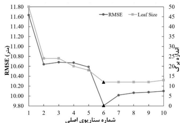
شکل ۱۲- نمودار نتایج سناریوهای منتخب شماره ۱ تا ۱۰
