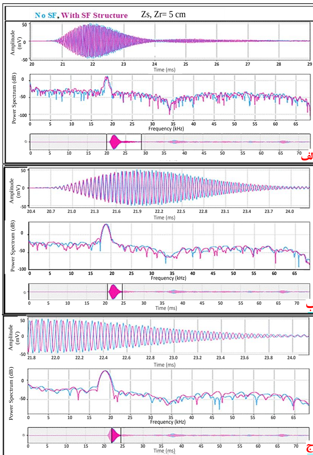
شکل ۲- الف) تغییر دامنه سیگنال‌های دریافتی مستقیم و بازتابی و توان طیفی سیگنال صوتی، ب) تغییر دامنه و توان پیشینه اول، ج) تغییر فاز و تاخیر در سیگنال مستقیم، در عمق ۵ سانتی متر. در غیاب (آبی) و در حضور انگشتان نمکی (صورتی).
