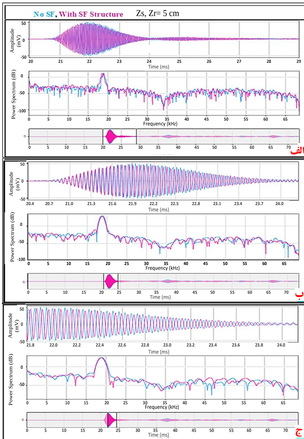
شکل ۲- الف) تغییر دامنه سیگنال‌های دریافتی مستقیم و بازتابی و توان طیفی سیگنال صوتی، ب) تغییر دامنه و توان پیشینه اول، ج) تغییر فاز و تاخیر در سیگنال مستقیم، در عمق ۵ سانتی متر. در غیاب (آبی) و در حضور انگشتان نمکی (صورتی).
