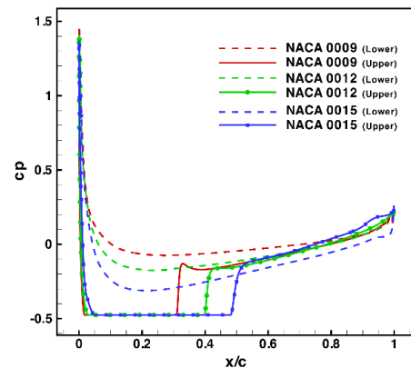
شکل ۱۴ - مقایسه ضریب فشار با افزایش ضخامت هیدروفوئیل‌های ۴ رقمی ناکا در عدد کاویتاسیون ۰/۵، زاویه حمله ۲/۵ درجه و عمق غرق‌شدگی ۰/۵ طول وتر هیدروفوئیل
