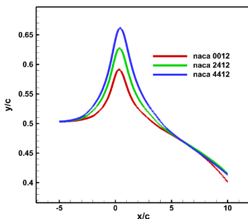
شکل ۱۵ - مقایسه شکل موج سطح آزاد با افزایش انحنا هیدروفوئیل‌های ۴ رقمی ناکا در عدد کاویتاسیون ۰/۵، زاویه حمله ۲/۵ درجه و عمق غرق‌شدگی ۰/۵ طول وتر هیدروفوئیل
