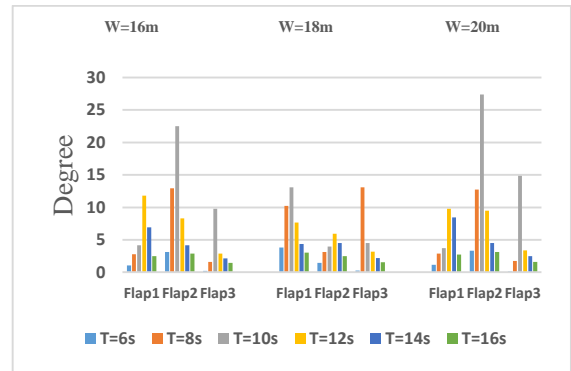
شکل ۱۵- تاثیر پهناي فلپ روی توان توليدي مبدلهاي انرژی
