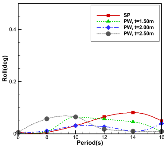
شکل ۱۹- تاثیر تغییر ضخامت فلپها
