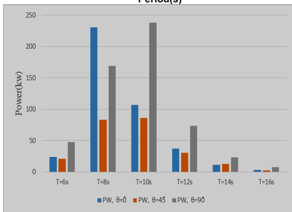
شکل ۲۶- تاثیر زاویه برخورد موج روی توان مبدل های انرژی
