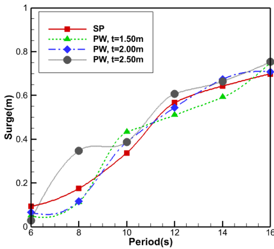
شکل ۱۴- تاثیر پهناي فلپ روی دامنه جابجاي فلپها تنها
