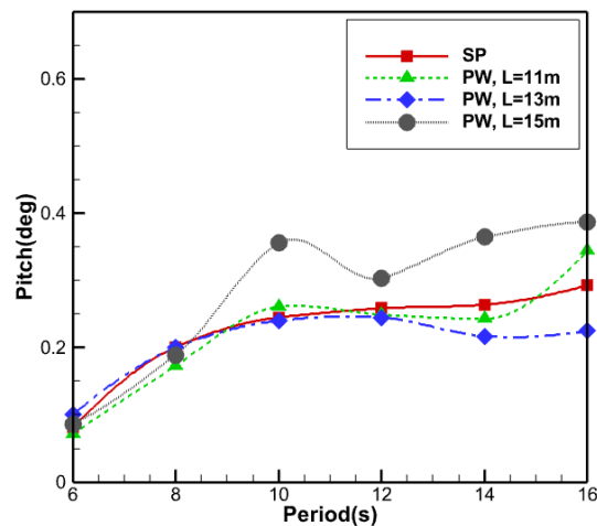
شکل ۷- تاثیر ارتفاع فلپ روی دامنه پیچ سکوی ترکیبی و سکوی تنها
