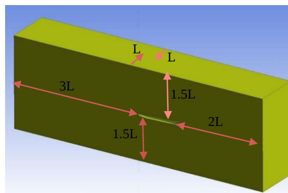
شکل ۲- دامنه محاسباتی مورد مطالعه
