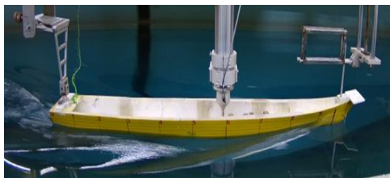
شکل ۶ - نمای مدل حین انجام تست کشش
