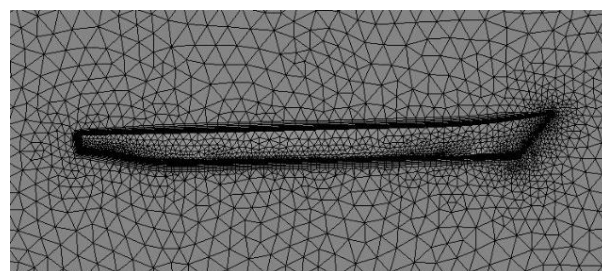
شکل ۱- شبکه‌بندی هندسه شناور مورد نظر
