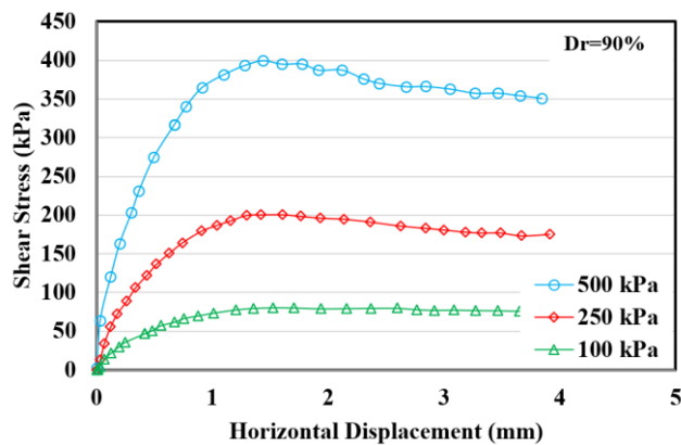
شکل ۷- نمودار تنش برشی - کرنش برشی برای ماسه کربناته با دانسیته نسبی ۹۰٪
