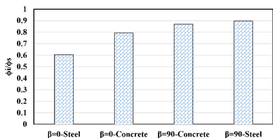
شکل ۲۴- تغییرات نسبت زاویه اصطکاک اندرکنش ماسه کربناته و صفحه فولادی و بتنی با توجه به زاویه برش به ماسه کربناته خالص برای ماسه کربناته با دانسیته نسبی ۹۰ درصد
