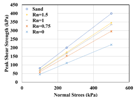
شکل ۱۵- پوش مقاومت برشی متناظر با تنش برشی ماکزیمم برای ماسه کربناته با دانسیته نسبی ۹۰٪ و صفحات فولادی با زبری مختلف
