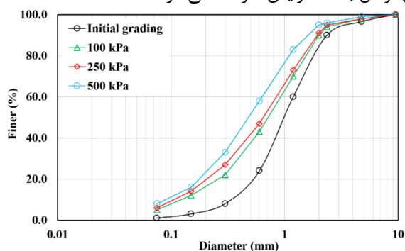
شکل ۲۵- منحنی دانه‌بندی مجدد برای ماسه کربناته در دانسیته نسبی ۳۰٪
